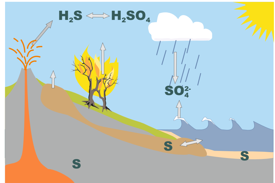
Svavlets kretslopp
