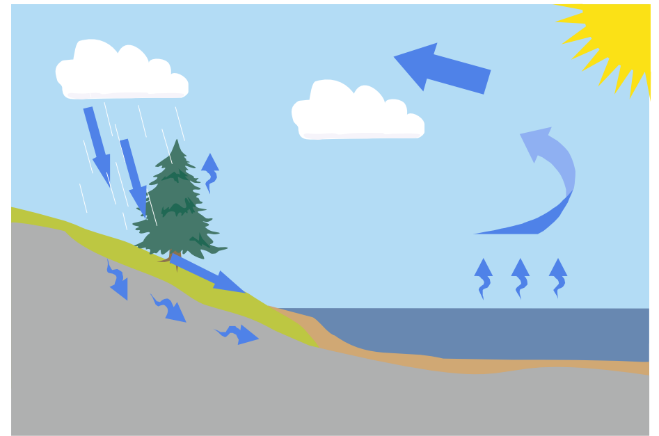
Vattnets kretslopp
