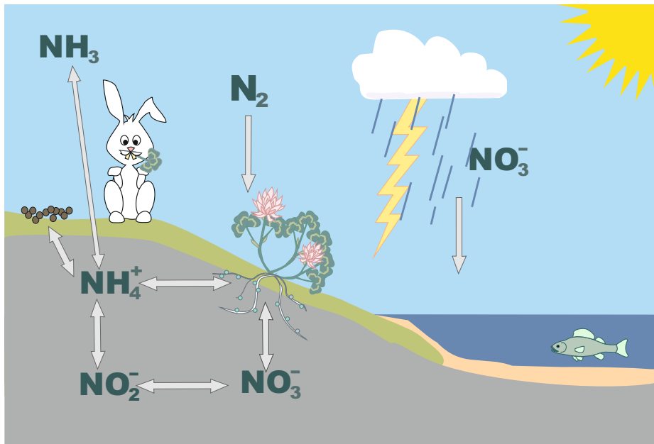
Kvävets kretslopp
