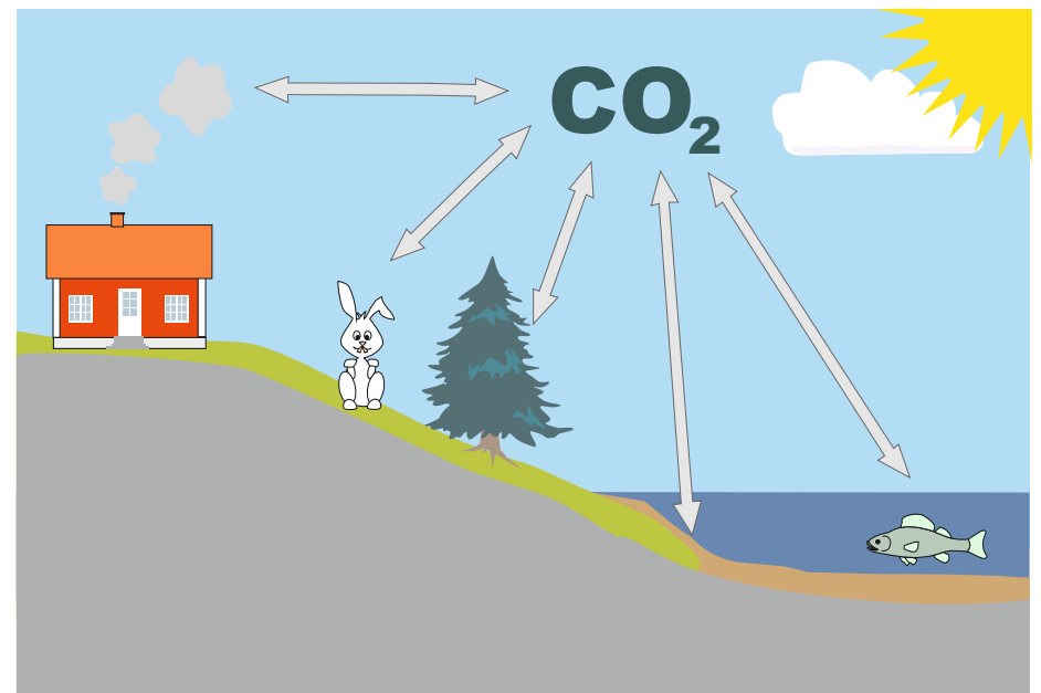
Kolets kretslopp
